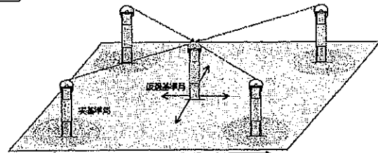
図1 仮想基準局方式によるカバレッジ
