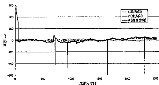
図 6 各座標成分の時系列変化
